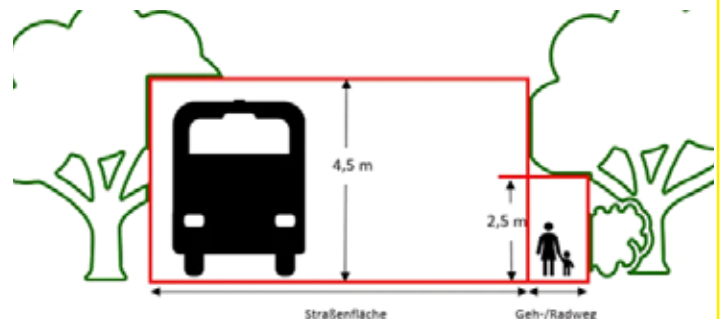
Lichttraumprofil: Der lichte Raum (innerhalb der roten Linie) muss lt. StVO freigehalten werden.
